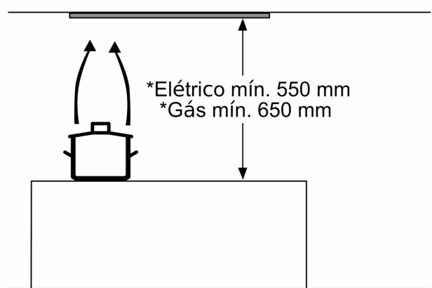
* a partir da aresta superior da grelha Medidas em mm
